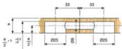
PERNO DE UNIÓN DOBLE
