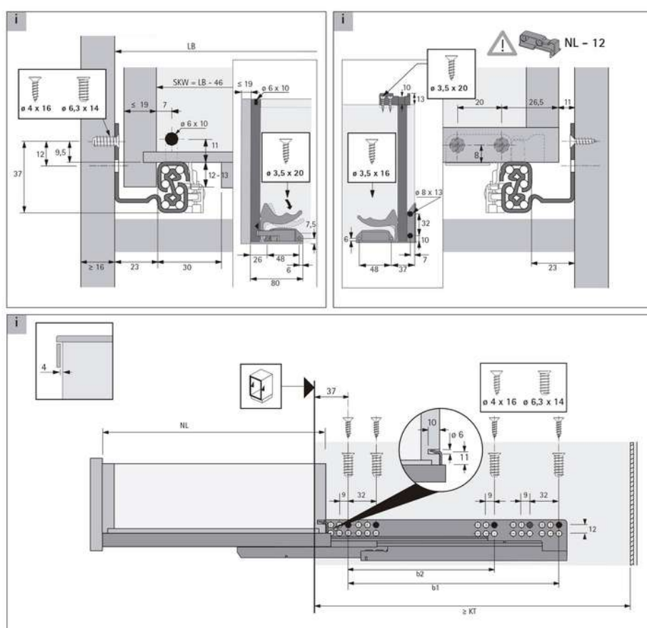
QUADRO V6 PUSH TO OPEN EB20 SIN TIRADOR
