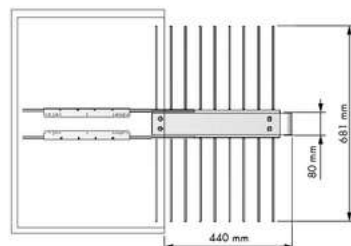
PANTALONERO DOBLE EXTRAÍBLE
