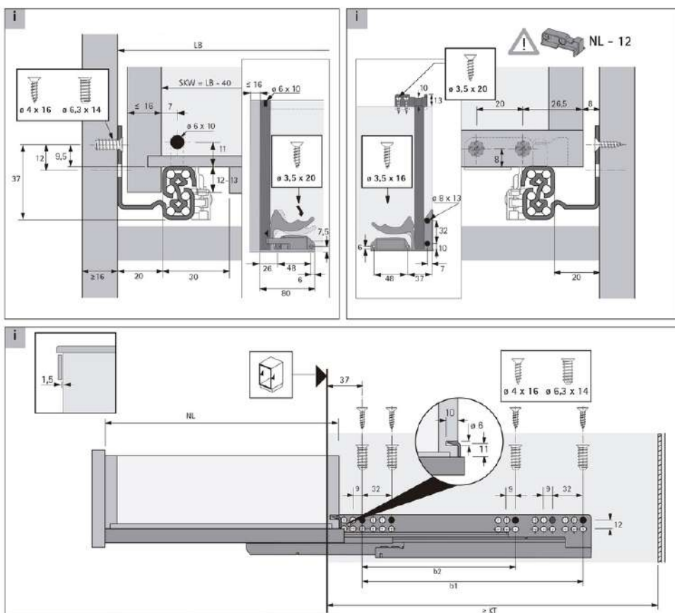
QUADRO V6 SILENT SYSSEM EB20 PARA TIRADOR
