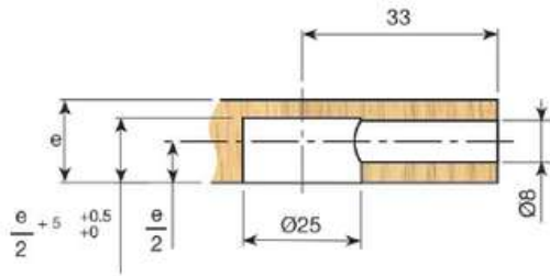
PERNO DE EXCÉNTRICA
