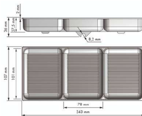
BANDEJA ACCESORIOS PANTALONERO
